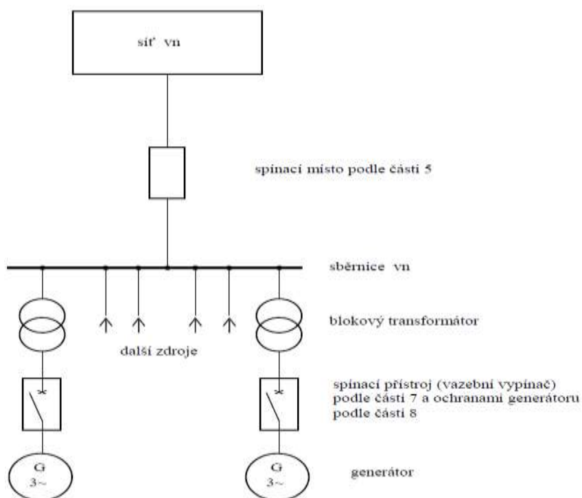
Příklad 7 Výrobna s více generátory v paralelním provozu se sběrní vn a decentralizovanými vypínači s ochranami.
