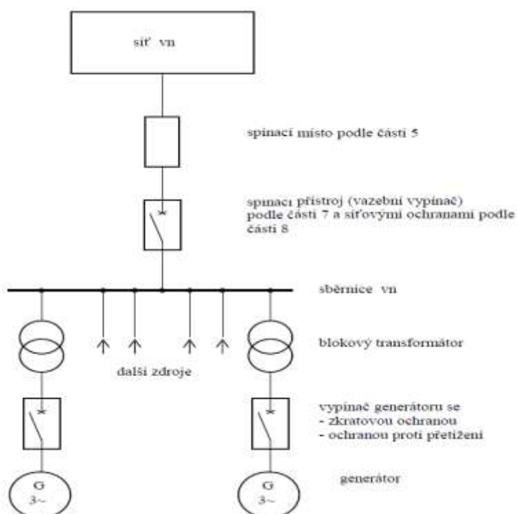
Příklad 8 Výrobna s více generátory v paralelním provozu se sítí bez možnosti ostrovního provozu, se sběrnicí vn a centrálním vypínačem s ochranami.
